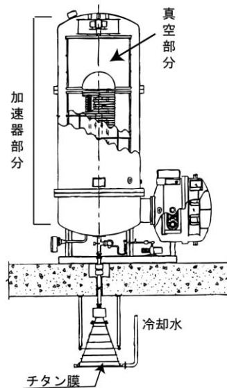
図1 電子線照射装置 (Natick 1957)
