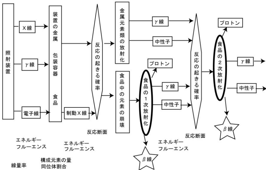
図7 計算に必要な要素
