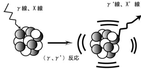
図8 X線γ線による励起
