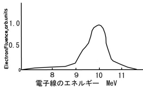
図6 10 MeV 電子線照射装置の電子線エネルギー分布 (Miller et al. : App. Radiat. Iso., 38, 507-512(1987))
