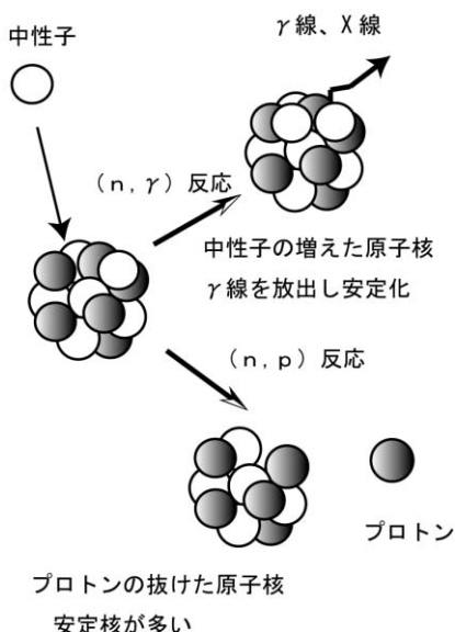
図12 中子と原子核との反応（中子捕獲反応） これは原子炉関連の防護対策として重要なために、研究が進んでいる。
