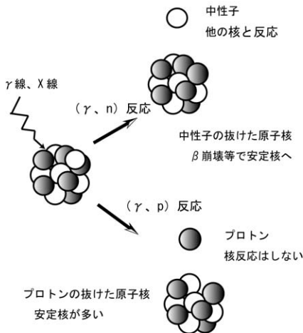
図9 X線γ線による中性子・プロトンの放出
