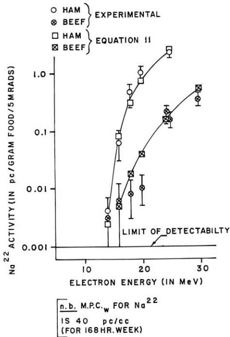
図4 照射食品中の Na22 の実測値と計算値(文献 8) 12MeV ~ 24MeV の電子線照射により Na23 ( \gamma, n ) Na22 の反応でできる。生成量とエネルギーとの関係を示している。
