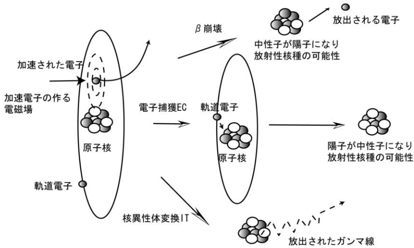
図10 電子線と核との作用
