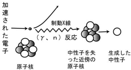
図11 制動放射 X線と中性子の放出
