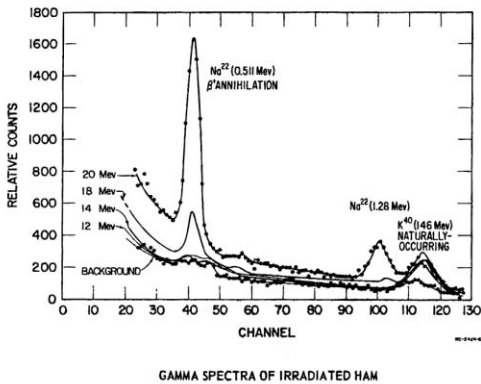
図 3 \gamma 線測定結果 (文献 9)
