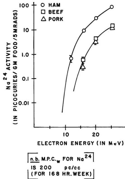
図5 照射食品中の Na24の実測値 (文献 9)
